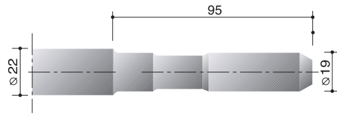
Shank: \varnothing 19 \times 95 \text{mm}
